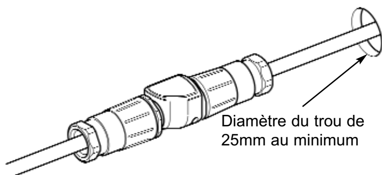
Fig. 8 – Passage de la connexion à travers la cloison
