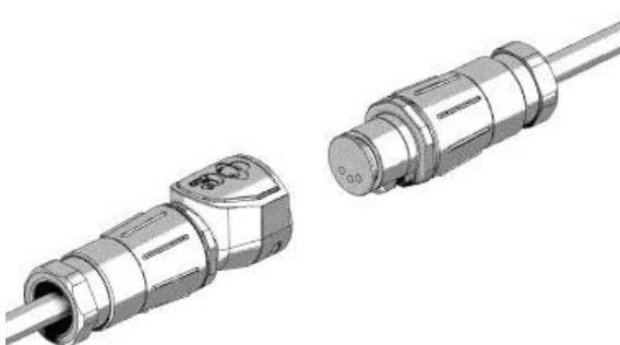
Fig. 9. Connexion de connecteurs Deutsch®
