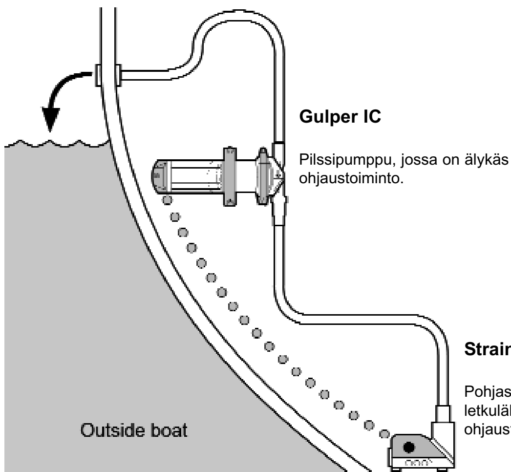
Kuva 1 -Tavallinen asennustapa: Gulper IC ohjattuna Strainer IC pohjasuodattimella
